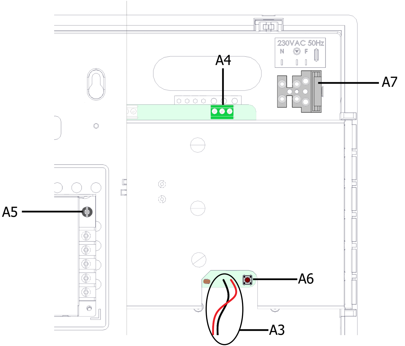
Şekil 4 Elektrik Bağlantıları
