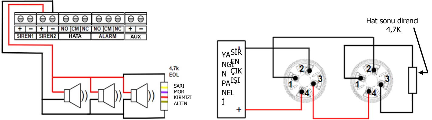
Şekil 6 Siren Bağlantısı
