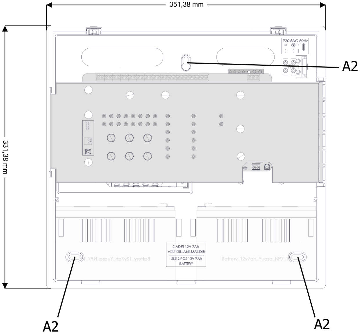
Şekil 3 Montaj Vida Delikleri
