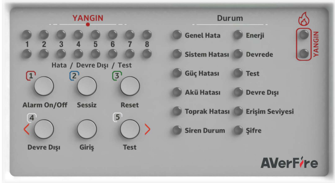
Kontrol Paneli Kullanıcı Arayüzü
