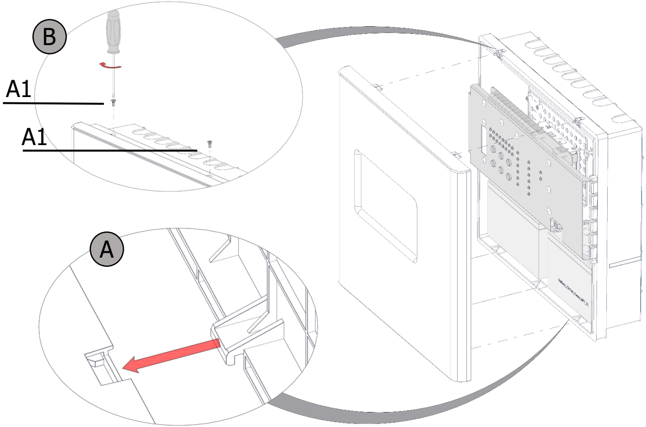
Şekil 2 Panel Ön Kapak Montajı
