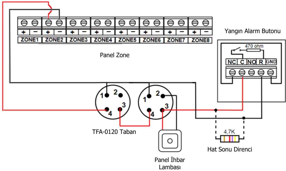
Şekil 7 Bölge Bağlantısı
